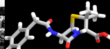
Molécula de Penicilina
